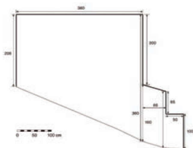
Prerez podzemnega hodnika pod cesto v Vincarje
